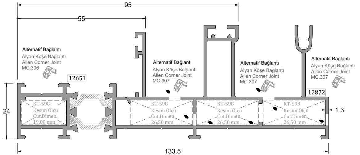
Tek Raylı Sineklikli Kasa Profili MONORAIL SCREENING FRAME PROFILE
