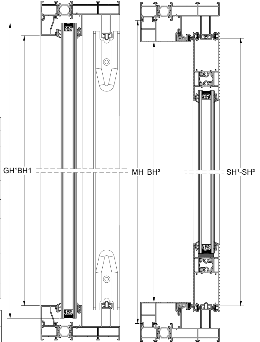
C-C KESİTİ
