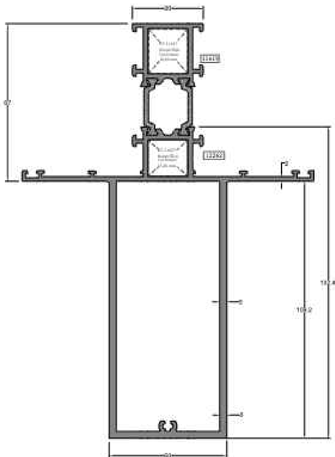
Ekstreyzeli Oturma Koltuğu Profili extruded seating chair profile
