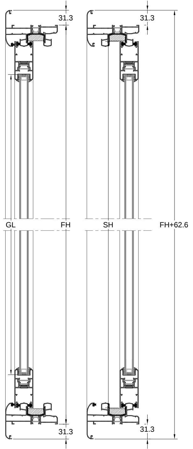
B-B KESİTİ
