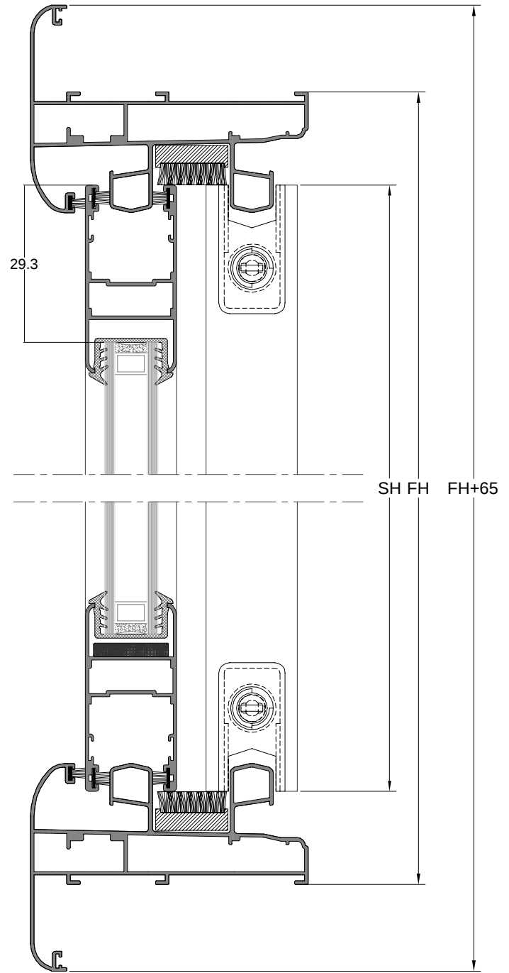
B-B KESİTİ
