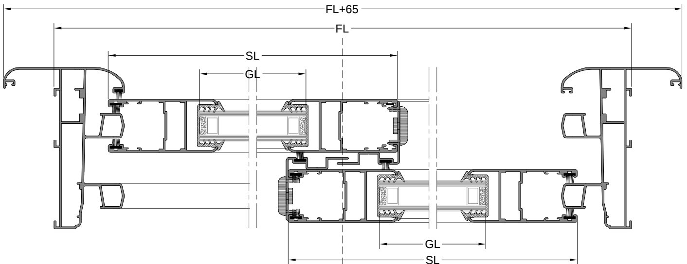
A-A KESİTİ
