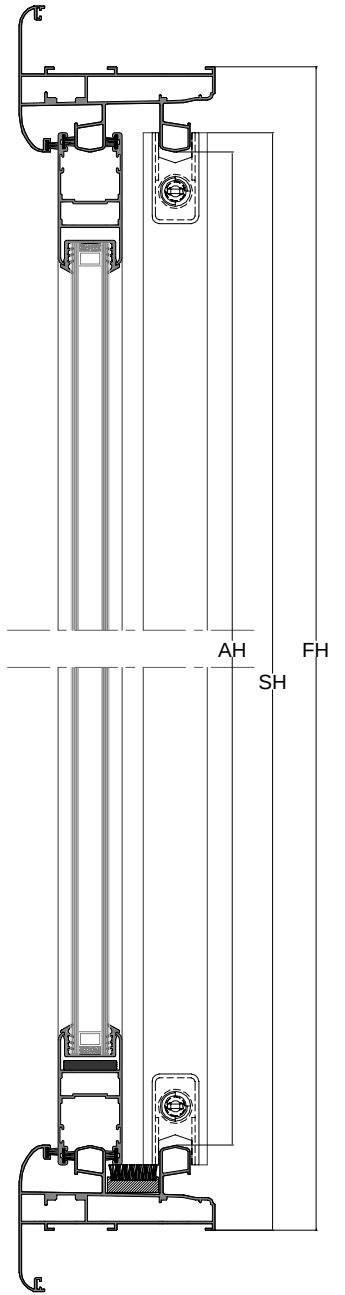
C-C KESİTİ
