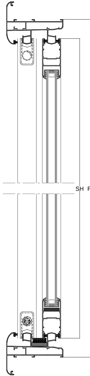
B-B KESİTİ
