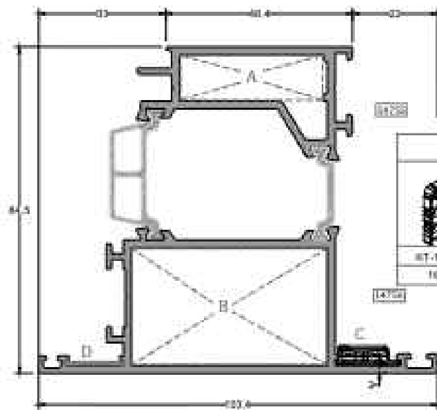
Diğer Açık Euro Kanatlı Kanat Profili Other Open Euro Winged Wing Profile
