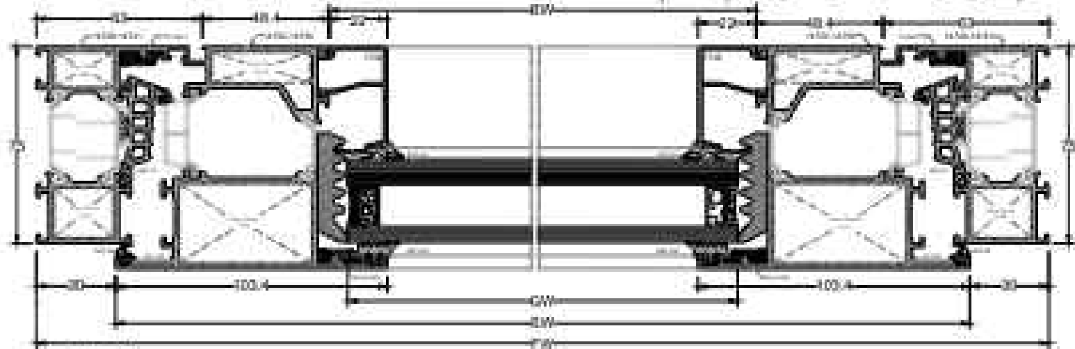
A-A KESİTİ
