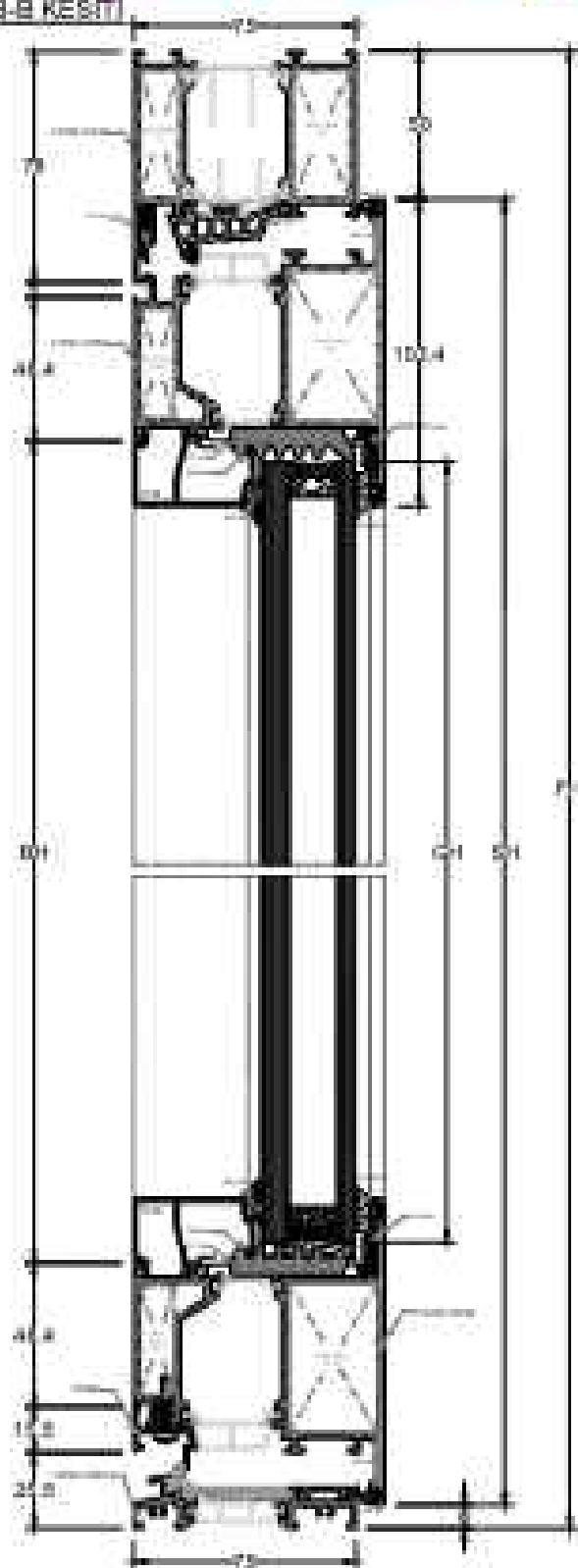
8-8 KESTI
