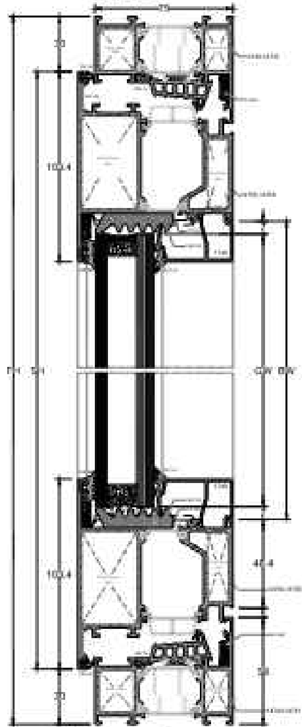
B-B KESİTİ
