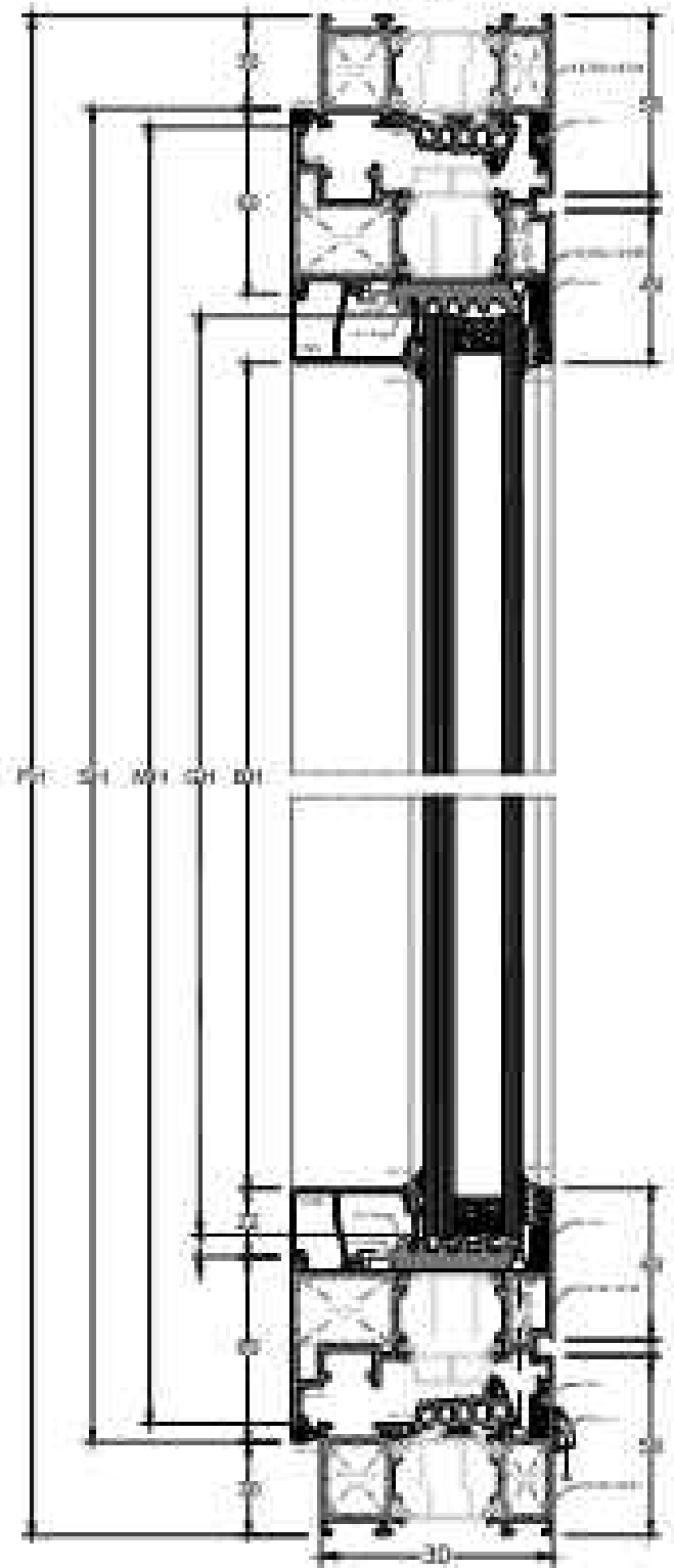
B-B KESİTİ
