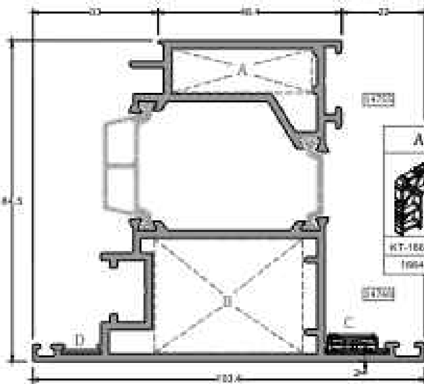
Diğer Açılır Pvc Kanallı Kanat Profili Other Opening PVC Channel Wing Profile
