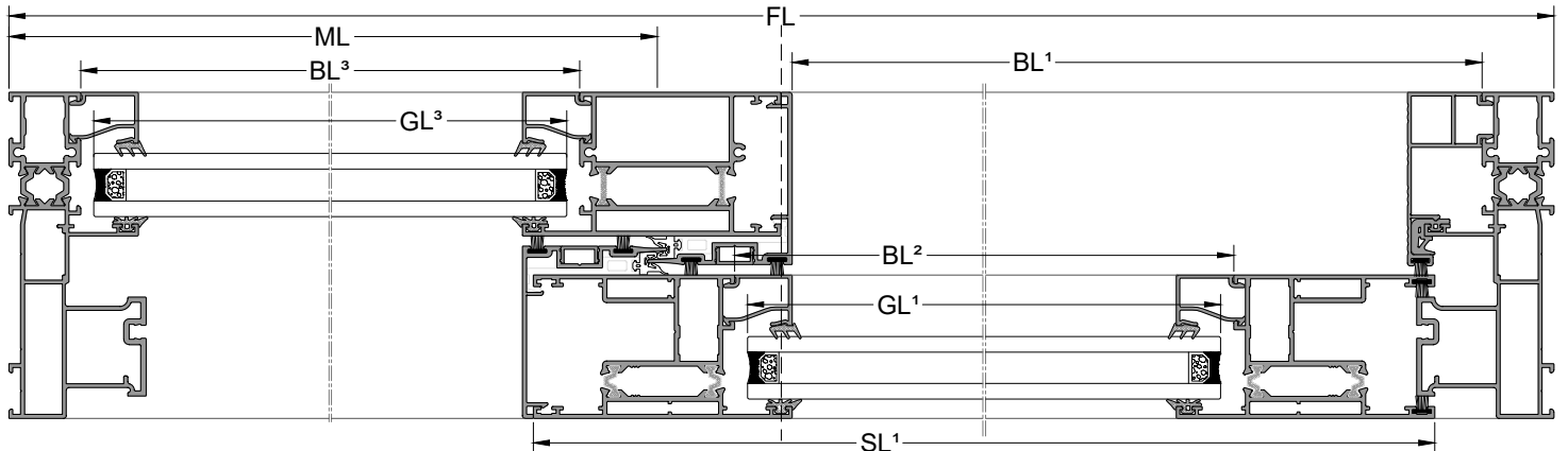
A-A KESİTİ
