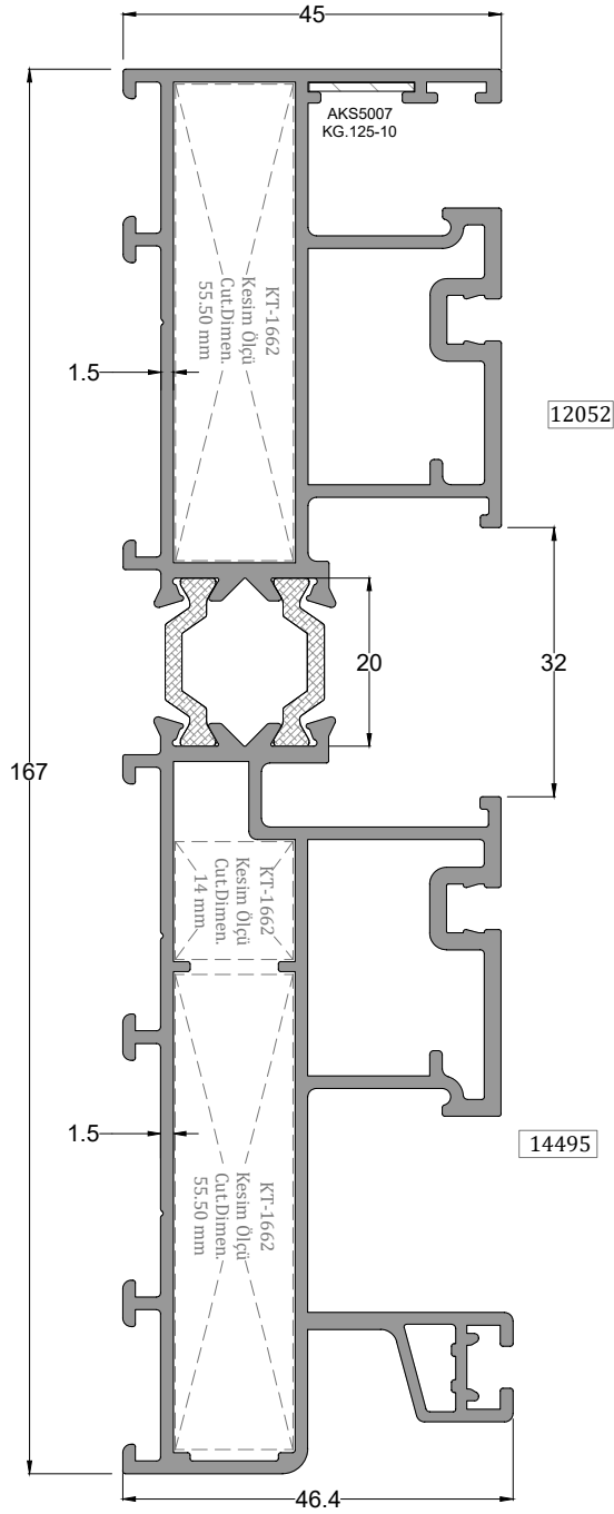
İki Raylı Sineklikli Kasa Profili DOUBLE RAIL SCREENING FRAME PROFILE
