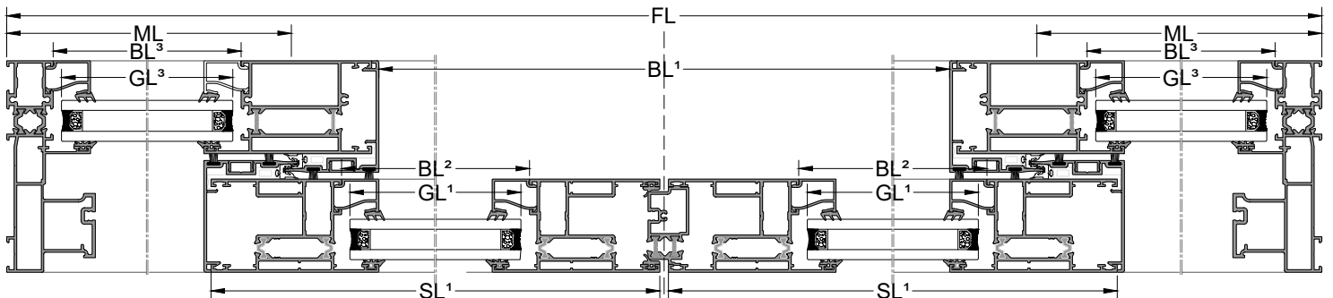
A-A KESİTİ
