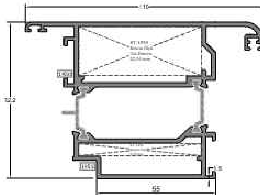
Diğer Açılır Kapanıl Profil Other Openable and Closeable Profile
