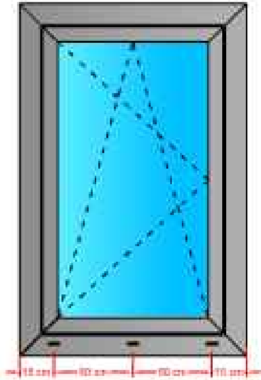
Su Tahliye İşlem Şeması WATER DRAINAGE PROCESS SCHEMATIC
