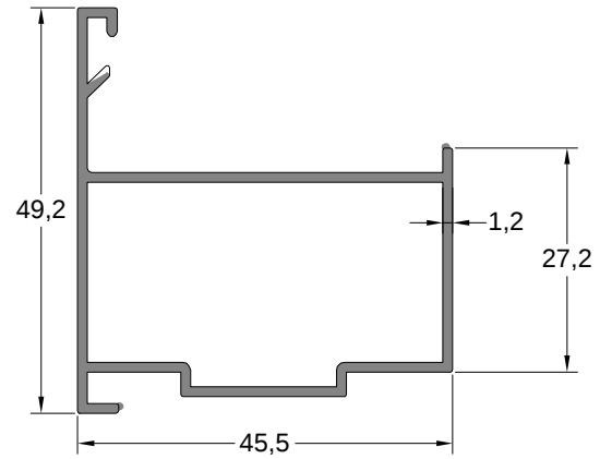
Pivot Adaptör Profili
