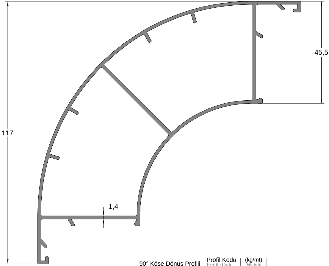
90° Köşe Dönüş Profili
