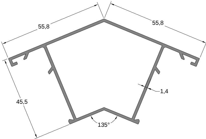
135° Köşe Dönüş Profili
